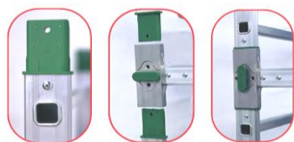
sistema di innesto traversa/fiancale con tirante di bloccaggio antisfilo
