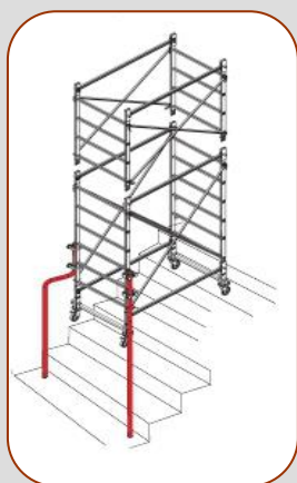
kit puntali per uso zoppo
