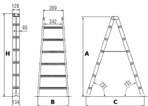
cerniere in fusione d'alluminio
